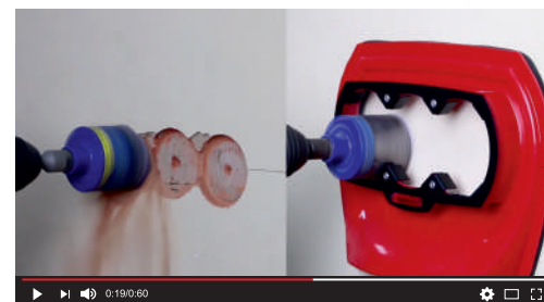
Направляющий коллектор для сверления подрозетников \varnothing 68, 72, 82
